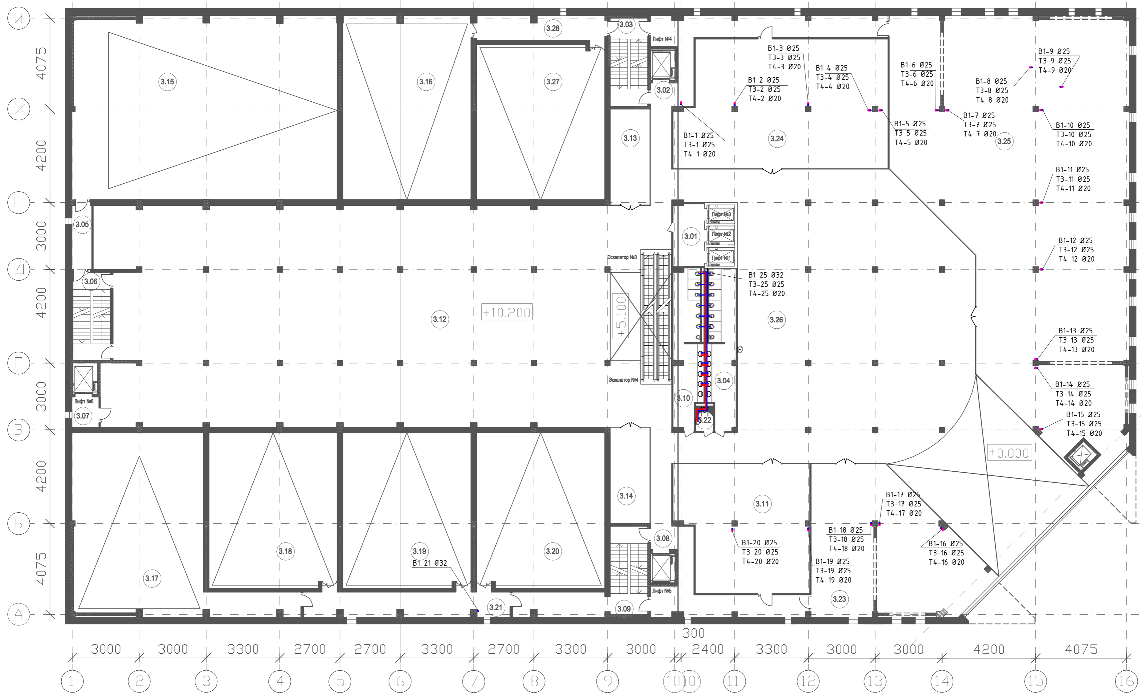
Экспликация помещений
