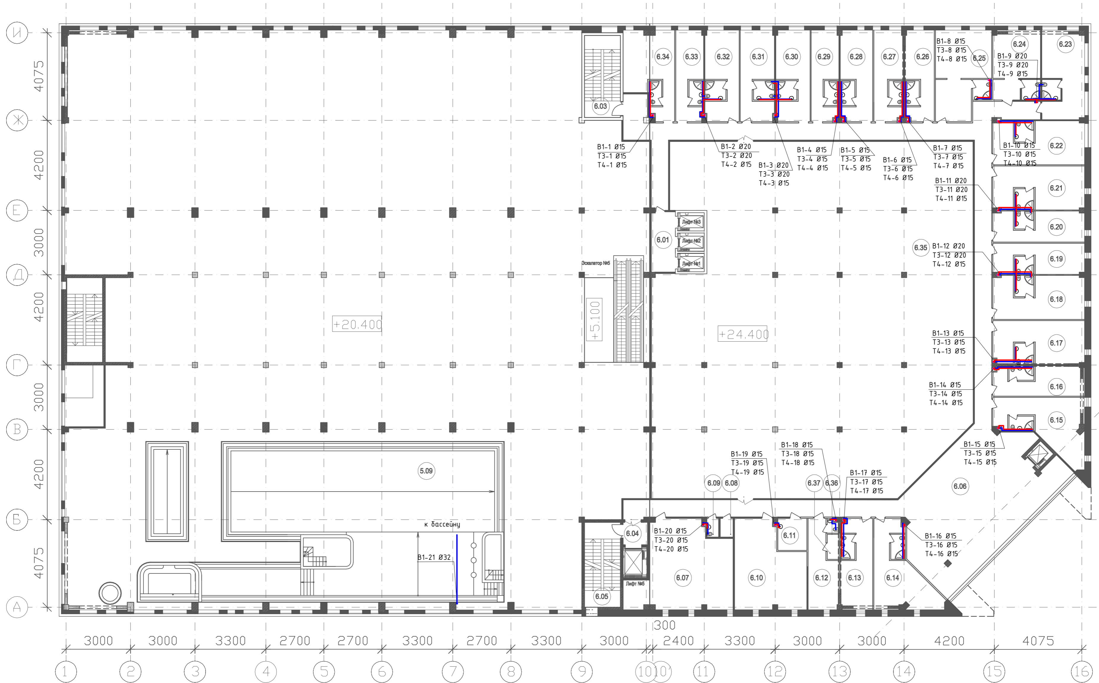
Экспликация помещений
