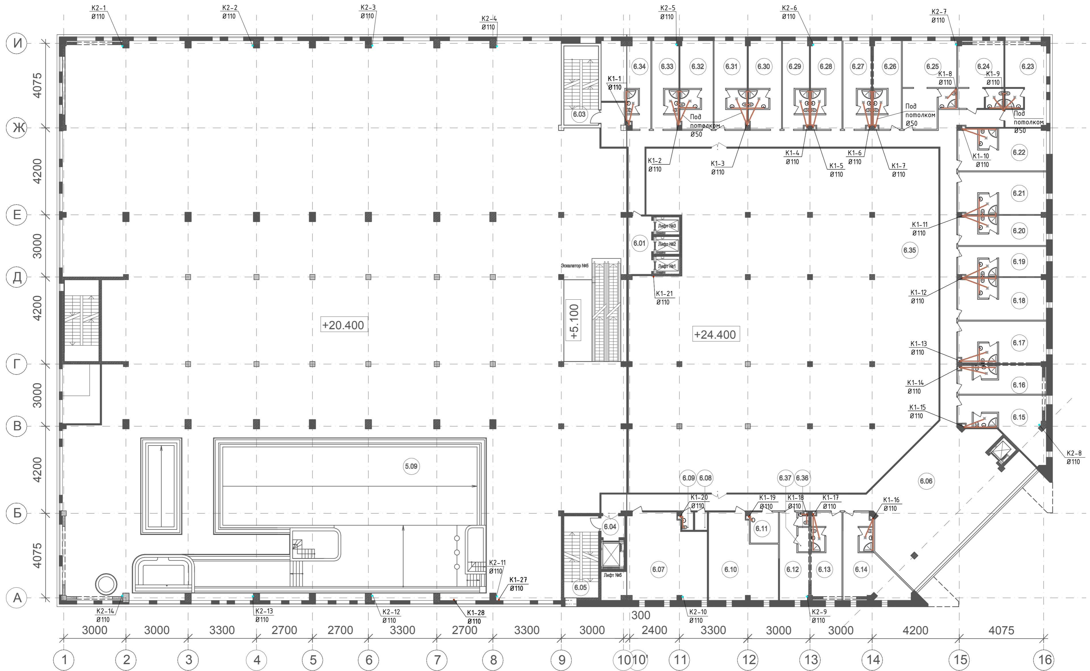
Экспликация помещений
